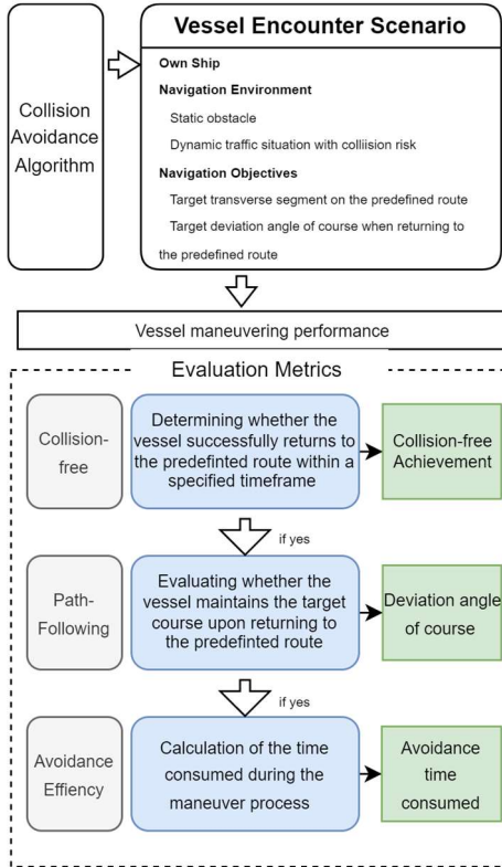
Fig. 1. Evaluation framework.
